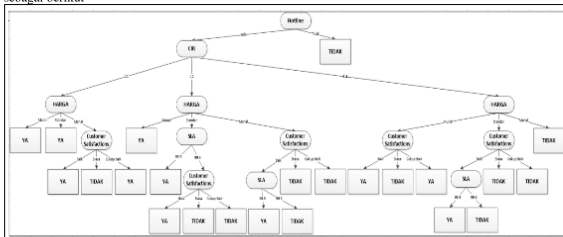
Gambar 5. Hasil Akhir Pembentukan Pohon Keputusan
