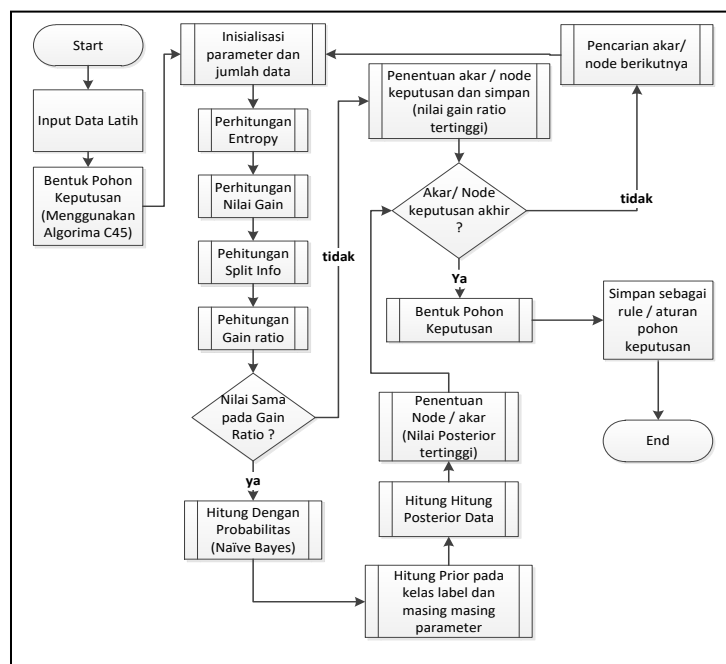
Gambar 2. Alur Pembentukan Pohon Keputusan Pemilihan ISP
