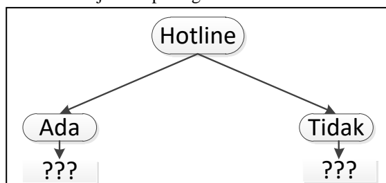
Gambar 3. Pembentukan Node Pertama Pohon Keputusan
