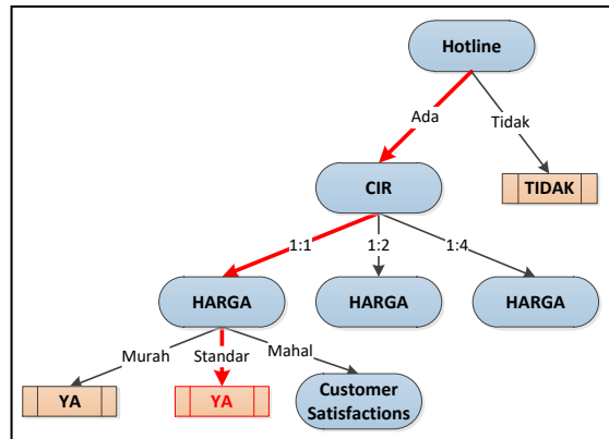
Gambar 6. Hasil Penelusuran Pohon Keputusan Pada Data Uji
